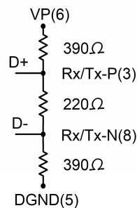
图 4 总线终端器
