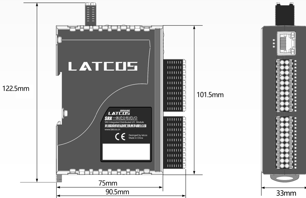
图 1 模块尺寸图
